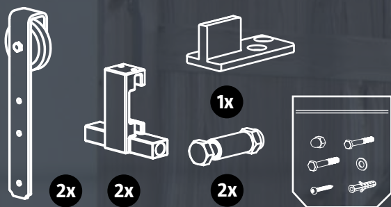
skład zestawu wózków
