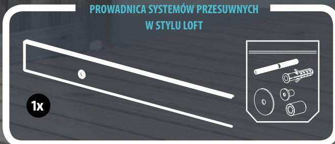
skład zestawu prowadnicy z mocowaniami
